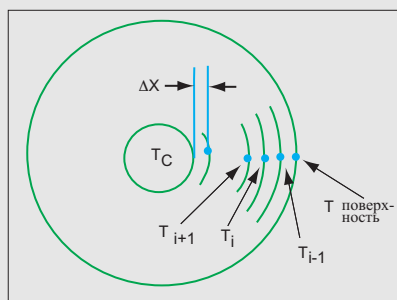
Компьютерное моделирование вулканизации резины
